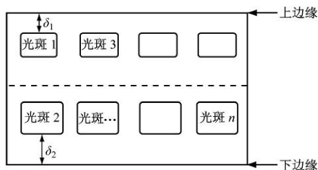
图 4 交替偏移聚焦策略
